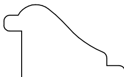
KL 21581 .781 x 1.281
